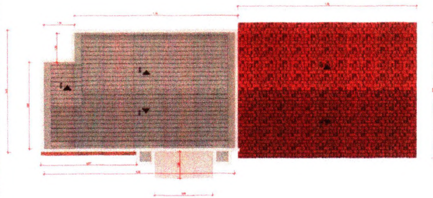
3 COBERTA ESCALA 1:50
