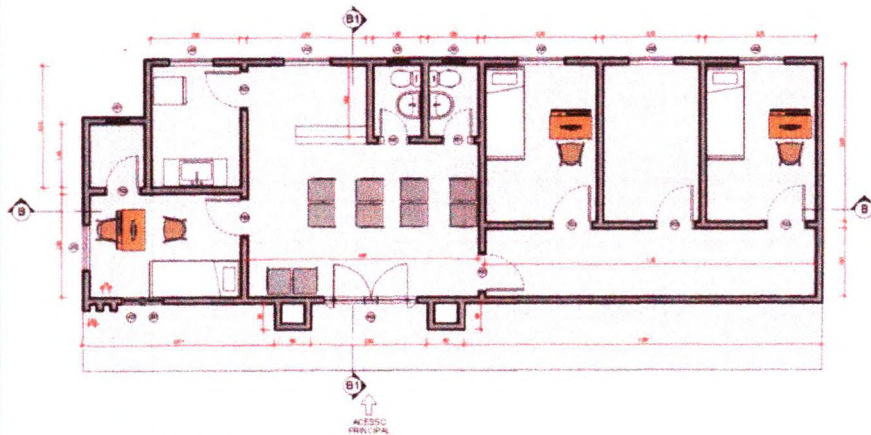
1 PLANTA NO TERRENO ESCALA 1:50
