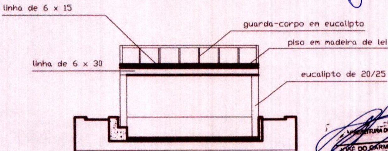
03 CORTE AA
