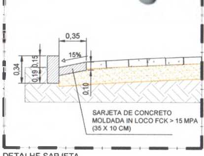
DETALHE SARJETA
