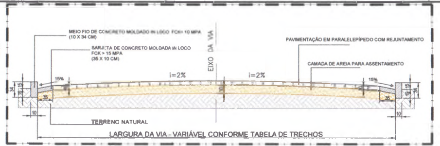
SEÇÃO TIPO - PAVIMENTAÇÃO EM PARALELEPÍEDO REJUNTADO - MEDIDAS EM CM
