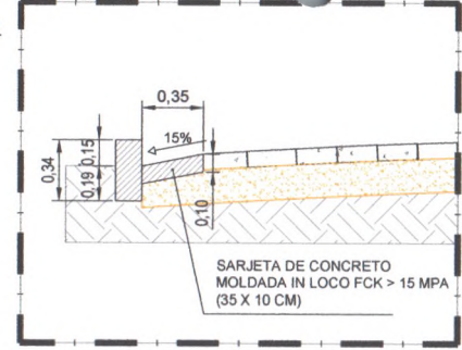
DETALHE SARJETA
