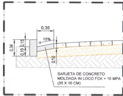
DETALHE SARJETA
