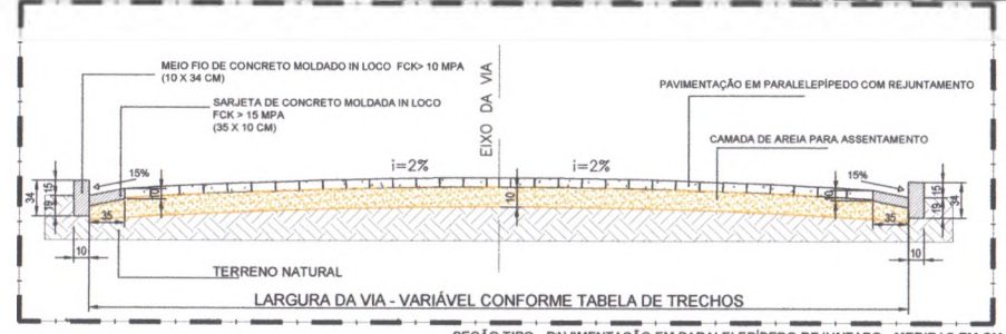
SEÇÃO TIPO - PAVIMENTAÇÃO EM PARALELEPÍPEDO REJUNTADO - MEDIDAS EM CM
