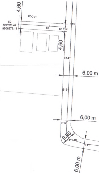
DETALHE SARJETA
