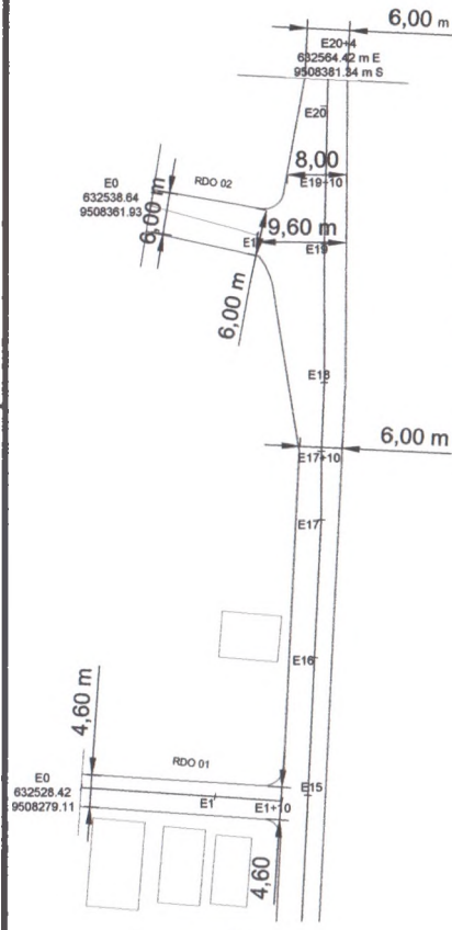
DETALHE SARJETA
