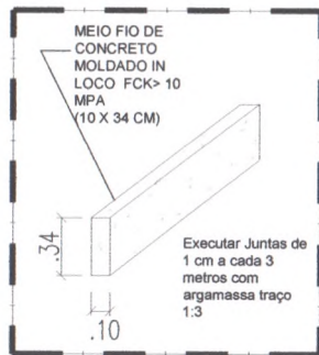
DETALHE BANQUETA/MEIO FIO
