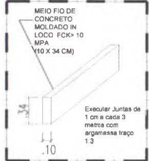
DETALHE BANQUET/MEIO FIO
